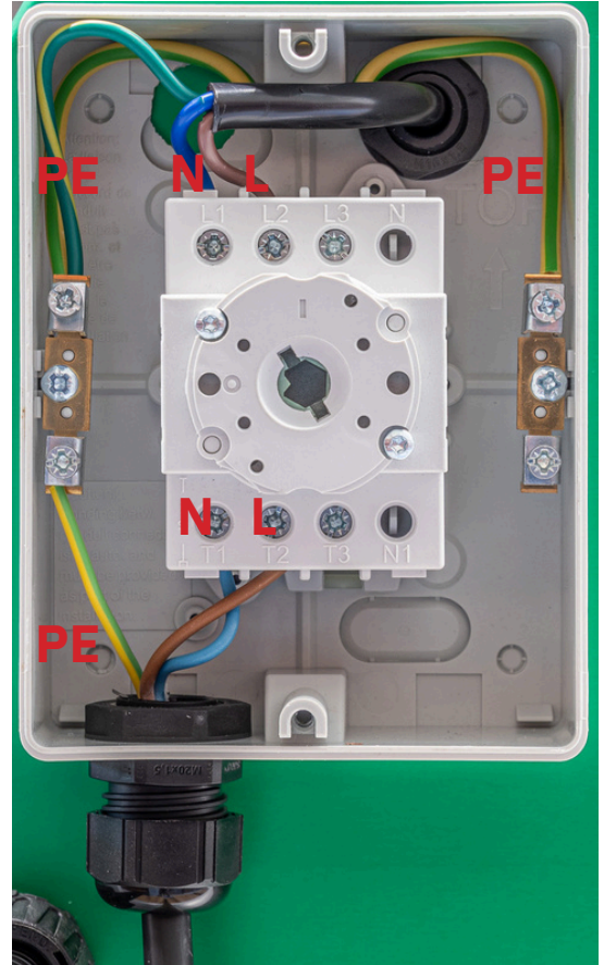
Después de la conexión del cable de alimentación se ha completado
