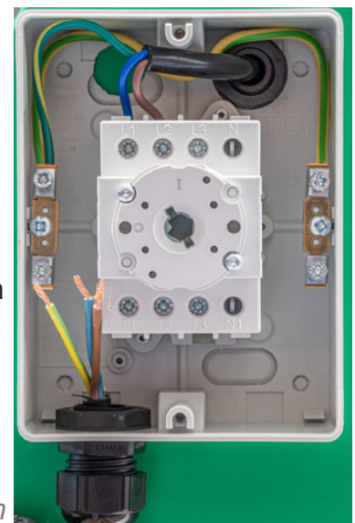
Cable de alimentación insertado, antes de la conexión
